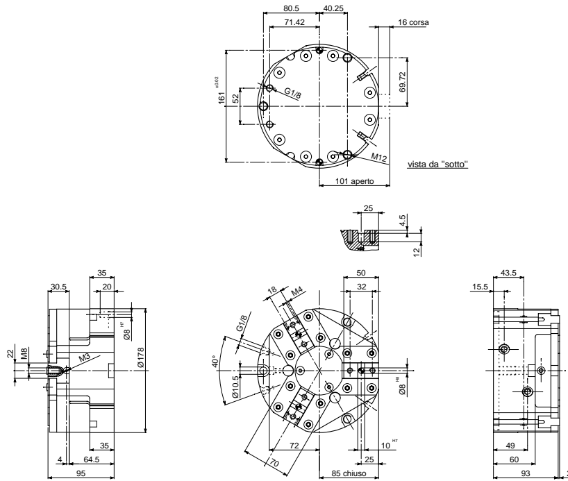
• Disegno QPG 317 • Drawing QPG 317 • Zeichnung QPG 317 • Dessin QPG 317
